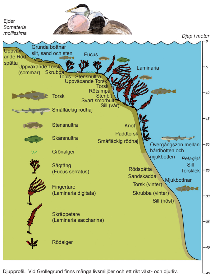
Djupprofil. Vid Grollegrund finns många livsmiljöer och ett rikt växt- och djurliv. Illustration: Magnus Karlsson och Peter Göransson.
